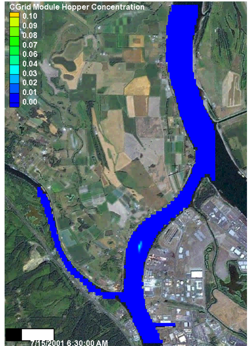
Hopper Dredge
